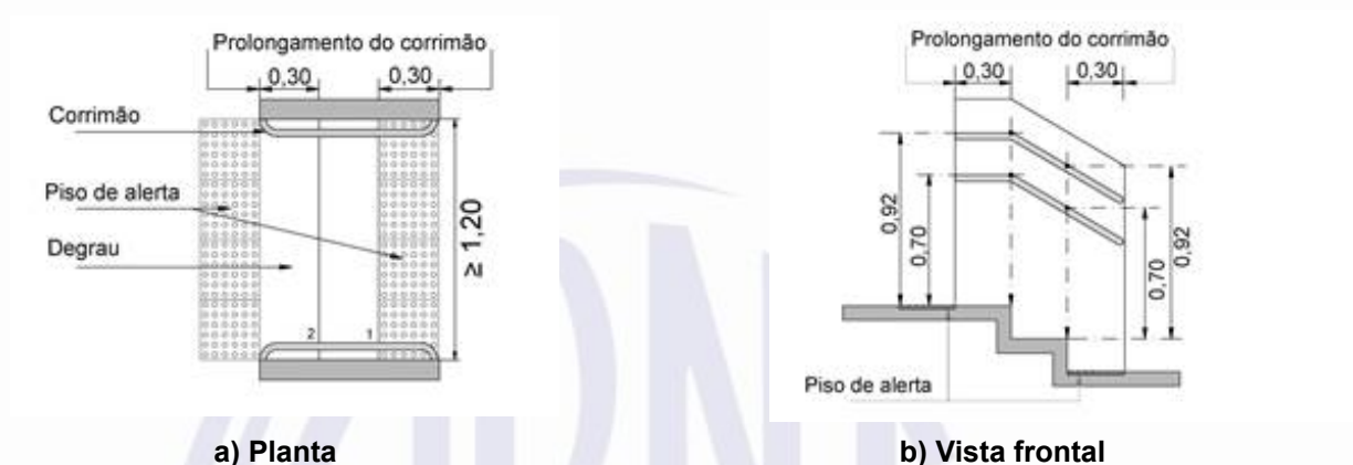
Figura 79 – Corrimão lateral em degrau isolado com dois degraus
